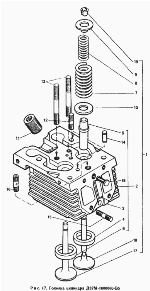
Рис. 17. Головка цилиндра ДЗ7М-1000080-Б5
